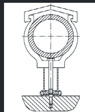
Távtartóval és fém profillal
