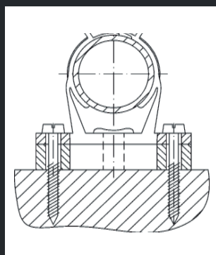
Csavarokkal és távtartóval
