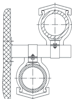
Ellentétes fém rögzítőelemmel egy fém profilon (függőleges vagy függő csőrögzéshez)
