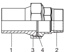
Rohrverschraubung PP-INDUSTRIAL-V2A mit Flachdichtung und Anschluss für Metallgewinde
