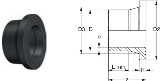
25.80.01.101 PE100 V-Bund kurz gerillt SDR11 schwarz PE100 Flange adaptor spigot short grooved SDR11 black
