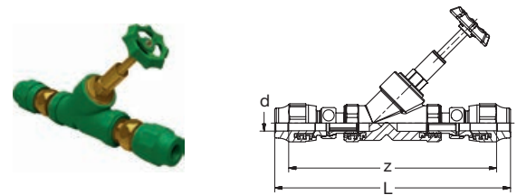
G 8655B PP-RCT-RG Ventil Schrägsitz mit Metallsitz verschraubt grün G 8655/1B PP-RCT-Bronze Valve angle with metal seat union-nuts green
