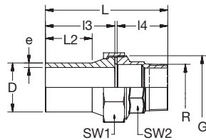
PP-INDUSTRIAL-V2A Ü-Verschraubung lang AG-keg Flachdichtring-EPDM 20°C/1.0MPa st SDR11 grau
