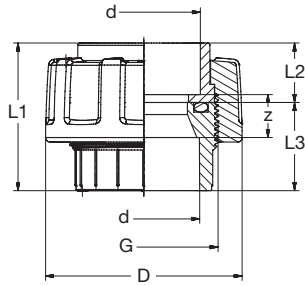
BG 8330A PP-INDUSTRIAL Verschraubung Runddichtring-EPDM grau PP-INDUSTRIAL Union O-Ring-gasket-EPDM grey
