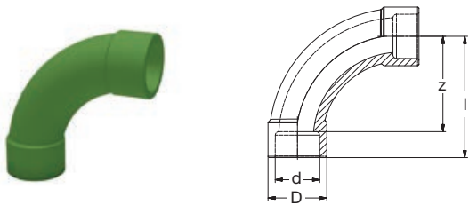
G 8002a PP-R Bogen 90° grün PP-R Bend 90° green
