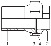
Rohrverschraubung PP-INDUSTRIAL-V2A mit Flachdichtung und Anschluss für Metallgewinde
