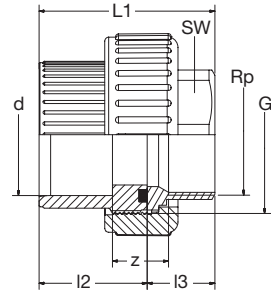
621.53.02 PVC-U-GJMW Ü-Verschraubung IG-zyl Flachdichtring-EPDM grau PVC-U-GJMW Transition-Union female-thread-cyl flat-gasket-EPDM grey
