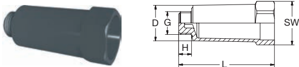
9900 Abpresszapfen AG-zyl mit NBR-Runddichtring Wall inlet plug male-thread-cyl with NBR-O-Ring gasket
