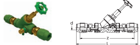
G 8650 PP-R-RG Ventil Schrägsitz mit Entleerung + Prüfstopfen verschraubt grün PP-R-Bronze Valve angle with drainage + test-plug and union-nuts green
