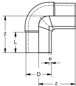
25.10.01.103 PE100 Winkel 90° lang SDR11 schwarz PE100 Elbow 90° long SDR11 black
