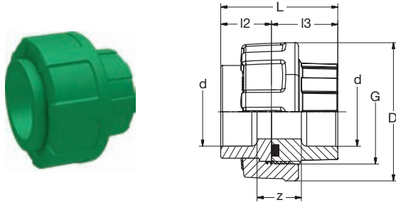
G 8330AB PP-RCT Verschraubung Runddichtring-EPDM grün PP-RCT Union O-Ring-gasket-EPDM green
