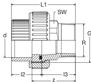
621.53.07 PVC-U-GJMW Ü-Verschraubung AG-keg Flachdichtring-EPDM grau PVC-U-GJMW Transition-Union male-thread-con flat-gasket-EPDM grey
