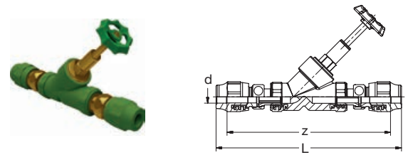
G 8655 PP-R-RG Ventil Schrägsitz mit Metallsitz verschraubt grün G 8655/1 PP-R-Bronze Valve angle with metal seat union-nuts green
