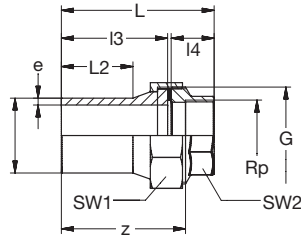
PP-INDUSTRIAL-V2A Ü-Verschraubung lang IG-zyl Flachdichtring-EPDM 20°C/1.0MPa st SDR11 grau
